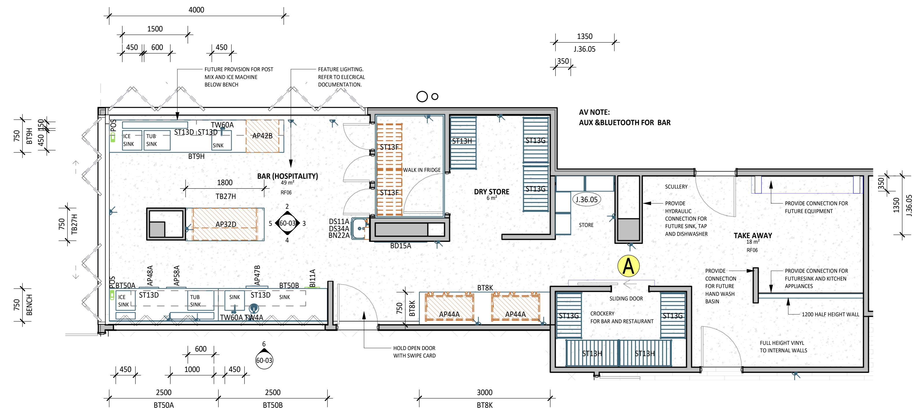
1 PLAN DETAIL 1 : 50
